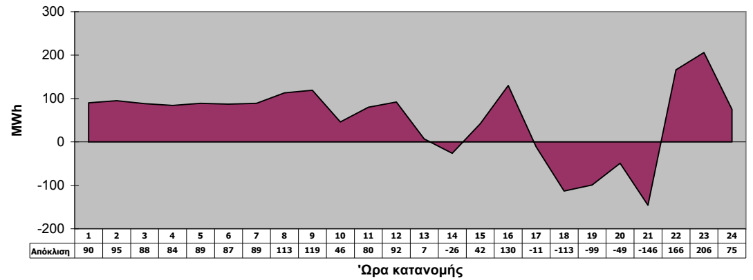
Υδροηλεκτρική Παραγωγή: Πραγματική - Δηλωθείσα Υποχρεωτική
