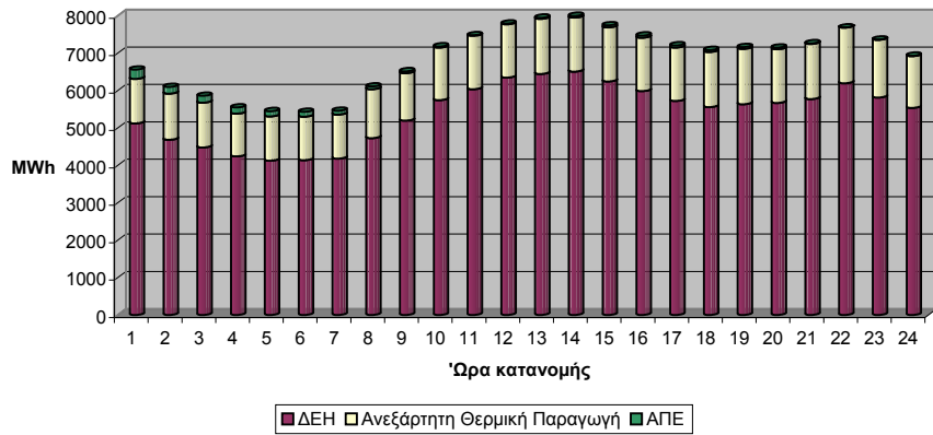
Μερίδιο ΔΕΗ: Πραγματική Λειτουργία
