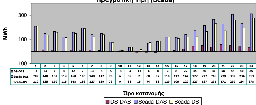
Αποκλίσεις Φορτίου: Δηλώσεις Φορτίου (DAS), Πρόβλεψη ΔΕΣΜΗΕ (DS), Πραγματική Τιμή (Scada)
