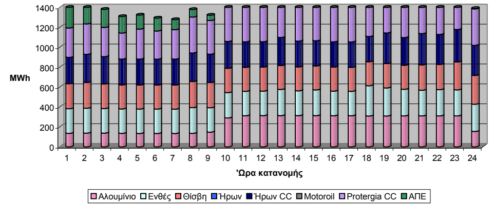
Ανεξάρτητη Παραγωγή: Πραγματική Λειτουργία
