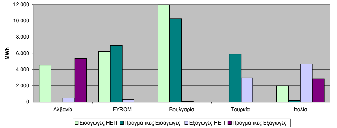
Εισαγωγές / Εξαγωγές ανά χώρα
