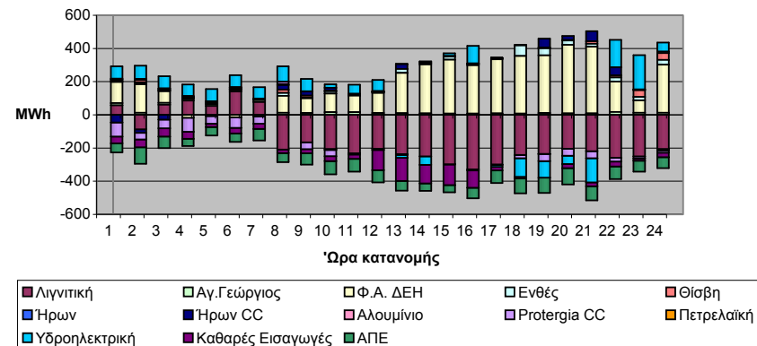
Μεταβολές Παραγωγής: Πραγματική Κατανομή - DS
