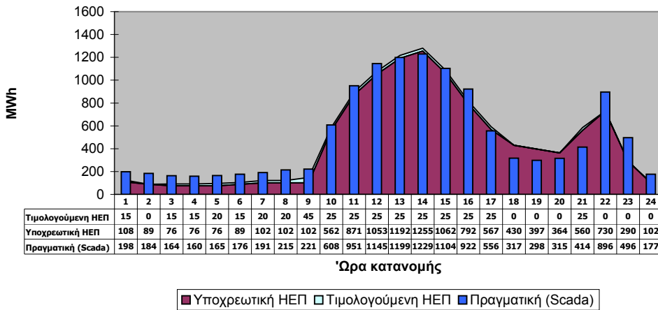
Υδροηλεκτρική Παραγωγή: ΗΕΠ, Πραγματική
