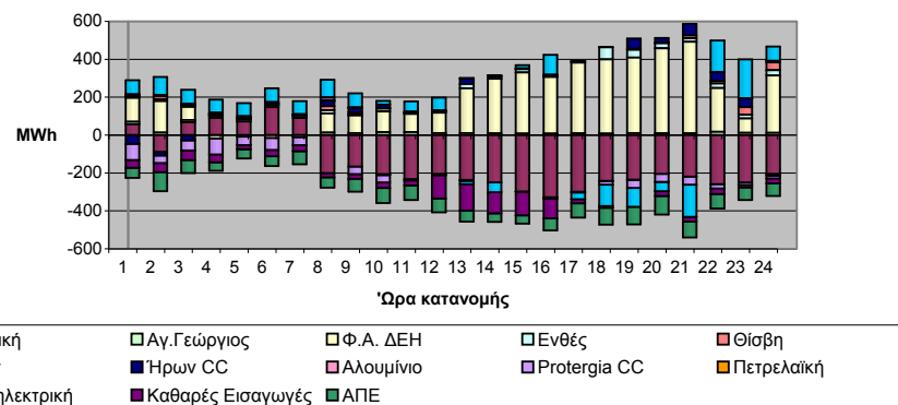
Μεταβολές Παραγωγής: Πραγματική Κατανομή - ΗΕΠ
