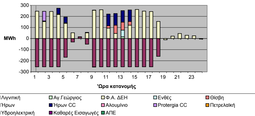
Μεταβολές Παραγωγής: Πρόγραμμα Κατανομής (DS) - ΗΕΠ
