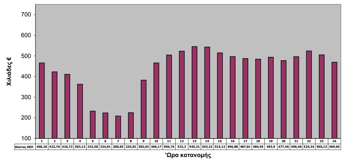
Ενεργειακό Κόστος: Επίλυση ΗΕΠ
