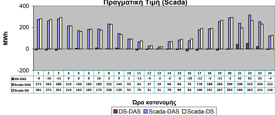
Αποκλίσεις Φορτίου: Δηλώσεις Φορτίου (DAS), Πρόβλεψη ΔΕΣΜΗΕ (DS), Πραγματική Τιμή (Scada)
