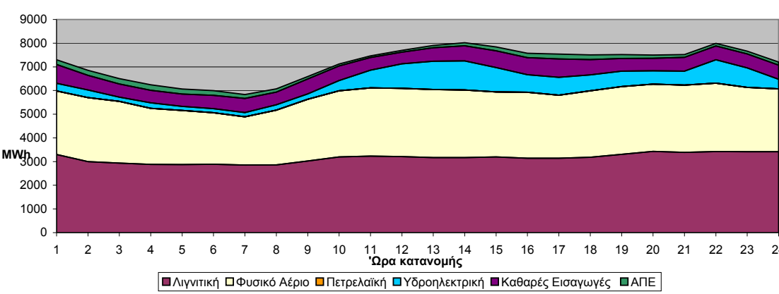
Πραγματική Παραγωγή ανά τεχνολογία
