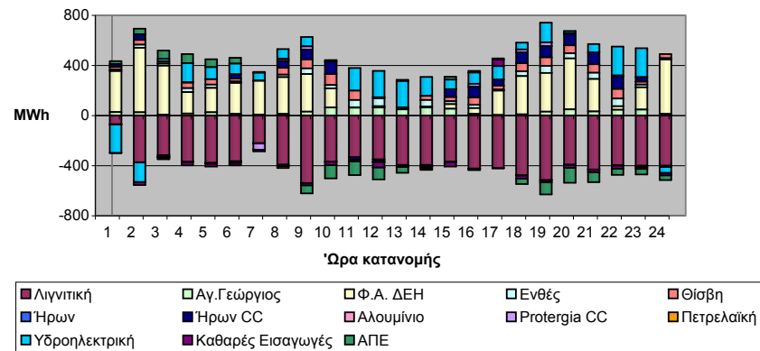
Μεταβολές Παραγωγής: Πραγματική Κατανομή - DS
