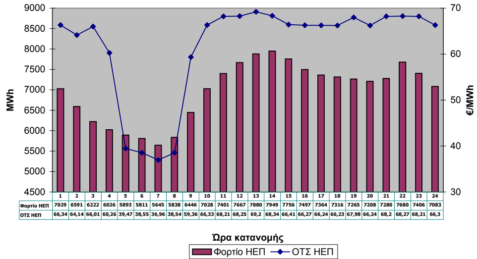
Φορτίο, Οριακή Τιμή Συστήματος: Επίλυση ΗΕΠ
