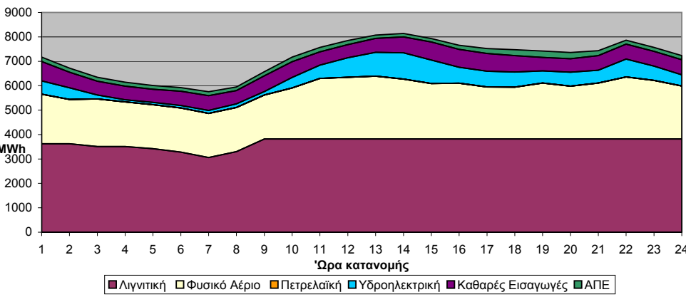
Παραγωγή ΗΕΠ ανά τεχνολογία
