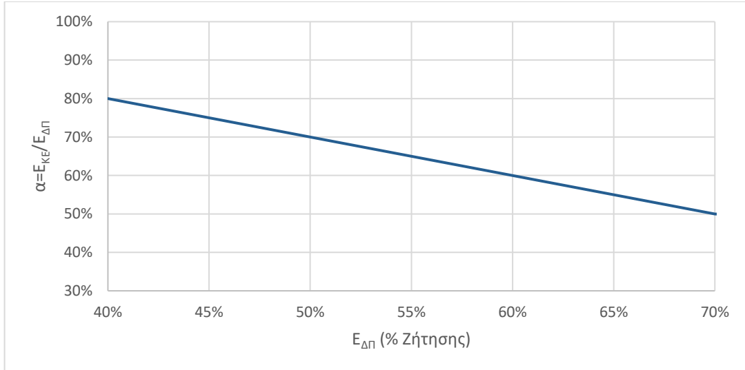
Σχήμα 1: Διάγραμμα ποσοστού Εγγυημένης Απορρόφησης ( \alpha_{εγγ} ) ως συνάρτηση της συνολικής ενέργειας Δηλώσεων Παραγωγής ( E_{\Delta\pi} )
