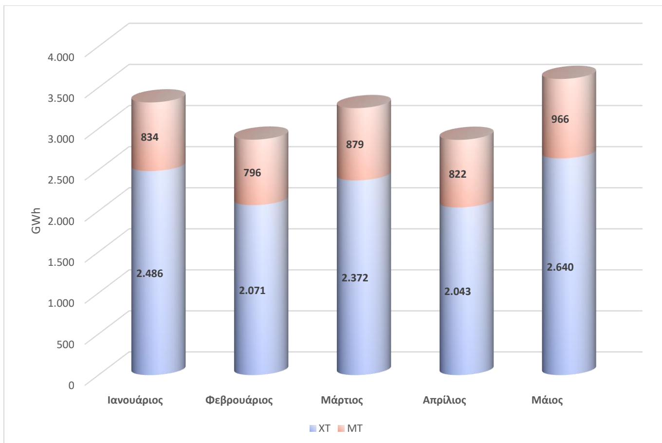
Σχήμα 8: Κατανάλωση ηλεκτρικής ενέργειας (GWh) ανά κατηγορία τάσης, Ιανουάριος – Μάιος 2023, (Πηγή: Ενημέρωση ΡΑΑΕΥ από ΔΕΔΔΗΕ ΑΕ)
