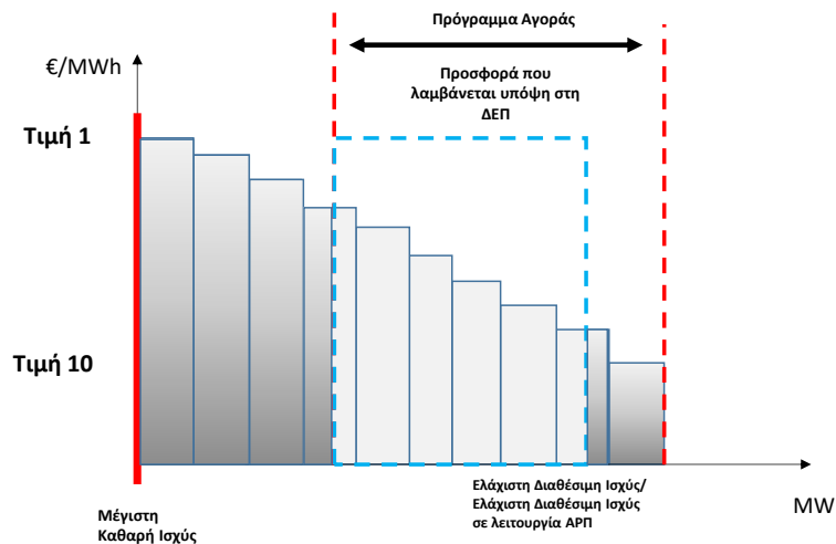
ΣΧΗΜΑ 317: ΚΑΘΟΔΙΚΗ ΠΡΟΣΦΟΡΑ ΕΝΕΡΓΕΙΑΣ ΕΞΙΣΟΡΡΟΠΗΣΗΣ ΜΙΑΣ ΟΝΤΟΤΗΤΑΣ ΥΠΗΡΕΣΙΩΝ ΕΞΙΣΟΡΡΟΠΗΣΗΣ
