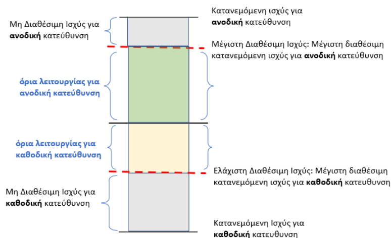
ΣΧΗΜΑ 7: ΟΡΙΑ ΛΕΙΤΟΥΡΓΙΑΣ ΧΑΡΤΟΦΥΛΑΚΙΩΝ ΚΑΤΑΝΕΜΟΜΕΝΩΝ ΜΟΝΑΔΩΝ ΑΠΕ ΜΗ ΕΛΕΓΧΟΜΕΝΗΣ ΠΑΡΑΓΩΓΗΣ ΚΑΙ ΧΑΡΤΟΦΥΛΑΚΙΩΝ ΚΑΤΑΝΕΜΟΜΕΝΟΥ ΦΟΡΤΙΟΥ (ΕΞΑΙΡΕΙΤΑΙ Η ΑΝΤΛΗΣΗ)
