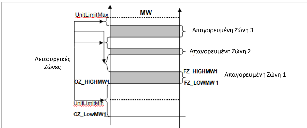
ΣΧΗΜΑ 28: ΑΠΑΓΟΡΕΥΜΕΝΗ ΖΩΝΗ ΣΤΙΣ ΚΑΤΑΝΕΜΟΜΕΝΕΣ ΥΔΡΟΗΛΕΚΤΡΙΚΕΣ ΜΟΝΑΔΕΣ ΠΑΡΑΓΩΓΗΣ
