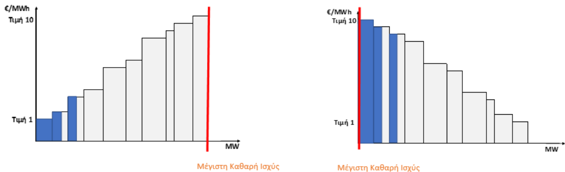
ΣΧΗΜΑ 13B ΠΑΡΑΔΕΙΓΜΑΤΑ ΒΗΜΑΤΙΚΩΝ ΠΡΟΣΦΟΡΩΝ ΑΝΟΔΙΚΗΣ (ΑΡΙΣΤΕΡΑ) ΚΑΙ ΚΑΘΟΔΙΚΗΣ (ΔΕΞΙΑ) ΕΝΕΡΓΕΙΑΣ ΕΞΙΣΟΡΡΟΠΗΣΗΣ ΓΙΑ ΧΑΡΤΟΦΥΛΑΚΙΑ ΚΑΤΑΝΕΜΟΜΕΝΟΥ ΦΟΡΤΙΟΥ ΠΟΥ ΑΦΟΡΟΥΝ ΑΝΤΛΗΣΗ
