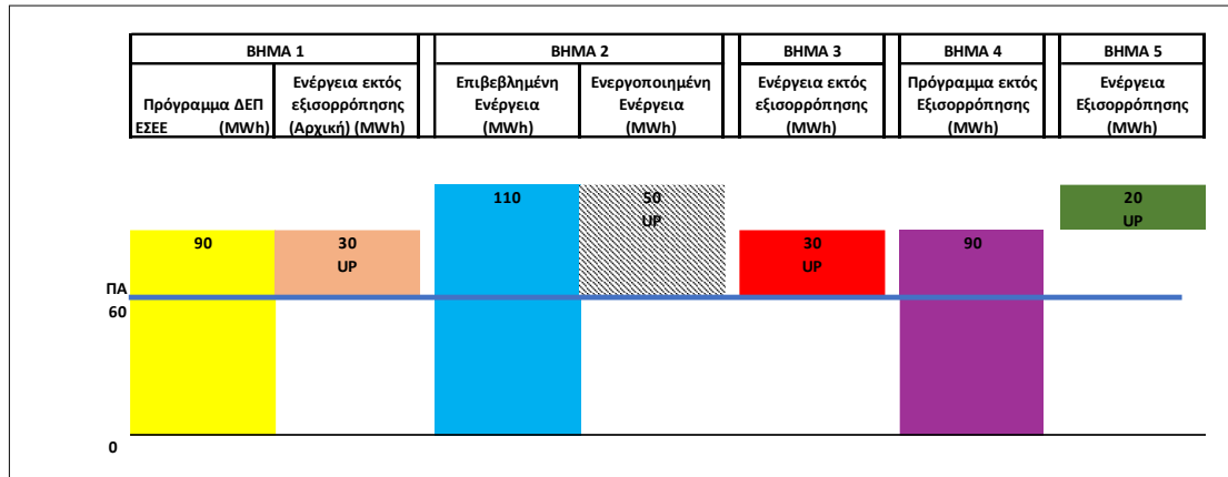
Σχήμα 15 Ενεργοποίηση ΔΕΠ ΕΣΣΕ προς την ίδια κατεύθυνση με τη συνολική ενεργοποιημένη ενέργεια χειροκίνητης ΕΑΣ (ανοδική) - Βήματα 1-5
