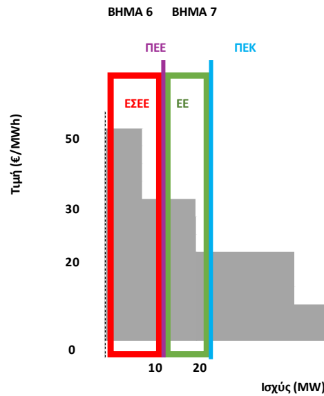
Σχήμα 33 Διάκριση ποσοτήτων στην καθοδική προσφορά χειροκίνητης ΕΑΣ - Βήματα 6-7
