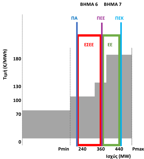
Σχήμα 16 Διάκριση ποσοτήτων στην ανοδική προσφορά χειροκίνητης ΕΑΣ - Βήματα 6-7
