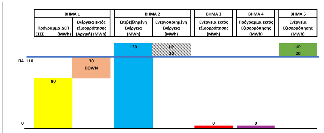
Σχήμα 19 Ενεργοποίηση ΔΕΠ ΕΣΕΕ προς την αντίθετη κατεύθυνση από τη συνολική ενεργοποιημένη ενέργεια - Βήματα 1-5
