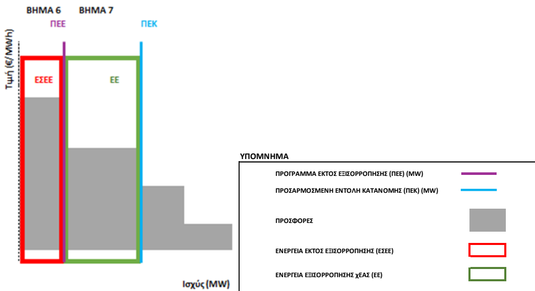
Σχήμα 5 Σχηματική αναπαράσταση των βημάτων 6-7 της μεθοδολογίας για καθοδική ενεργοποιημένη ενέργεια χειροκίνητης ΕΑΣ
