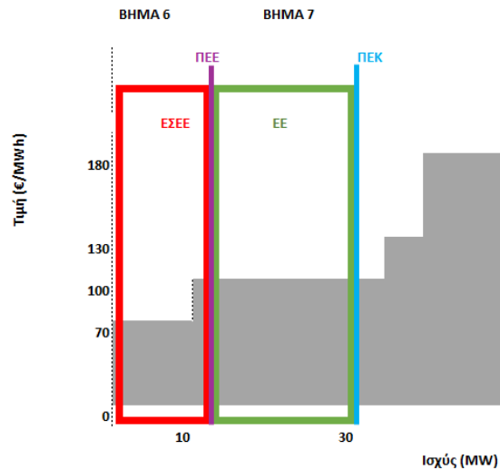
Σχήμα 31 Διάκριση ποσοτήτων στην ανοδική προσφορά χειροκίνητης ΕΑΣ - Βήματα 6-7
