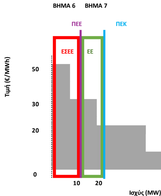
Σχήμα 29 Διάκριση ποσοτήτων στην καθοδική προσφορά χειροκίνητης ΕΑΣ - Βήματα 6-7
