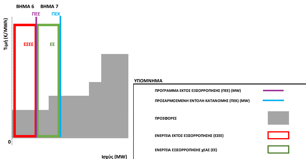
Σχήμα 7 Σχηματική αναπαράσταση των βημάτων 6-7 της μεθοδολογίας για ανοδική ενεργοποιημένη ενέργεια χειροκίνητης ΕΑΣ
