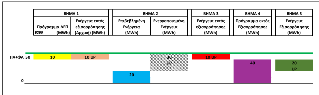
Σχήμα 30 Παράδειγμα με ανοδική ενεργοποιημένη ενέργεια για Χαρτοφυλάκιο Κατανεμόμενου Φορτίου - Βήματα 1-5
