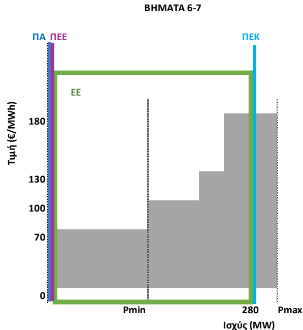
Σχήμα 24 Διάκριση ποσοτήτων στην ανοδική προσφορά χειροκίνητης ΕΑΣ - Βήματα 6-7
