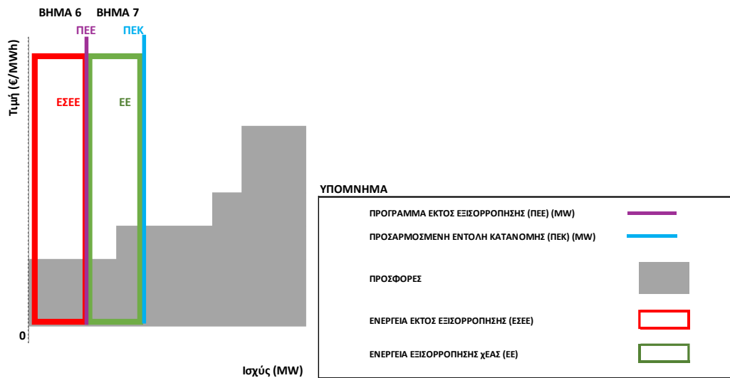
Σχήμα 4 Σχηματική αναπαράσταση των βημάτων 6-7 της μεθοδολογίας για ανοδική ενεργοποιημένη ενέργεια χειροκίνητης ΕΑΣ
