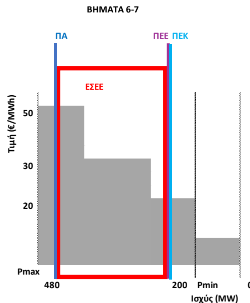
Σχήμα 22 Διάκριση ποσοτήτων στην καθοδική προσφορά χειροκίνητης ΕΑΣ - Βήματα 6-7
