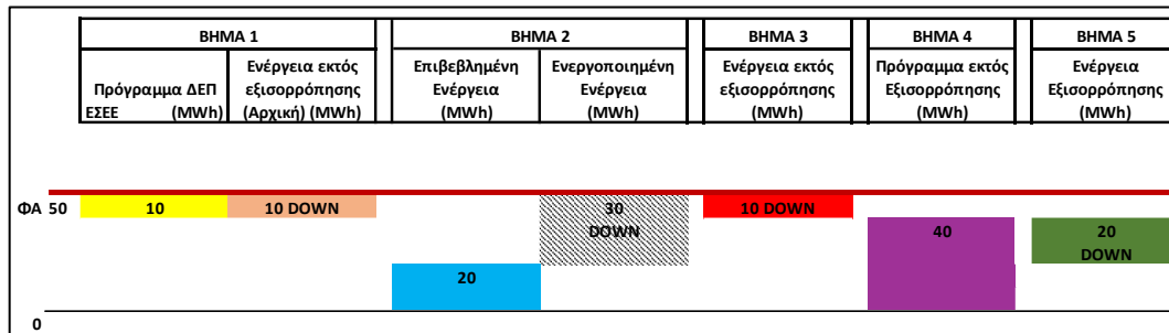
Σχήμα 28 Παράδειγμα με καθοδική ενεργοποιημένη ενέργεια για Χαρτοφυλάκιο Κατανεμόμενων Μονάδων ΑΠΕ Μη Ελεγχόμενης Παραγωγής - Βήματα 1-5
