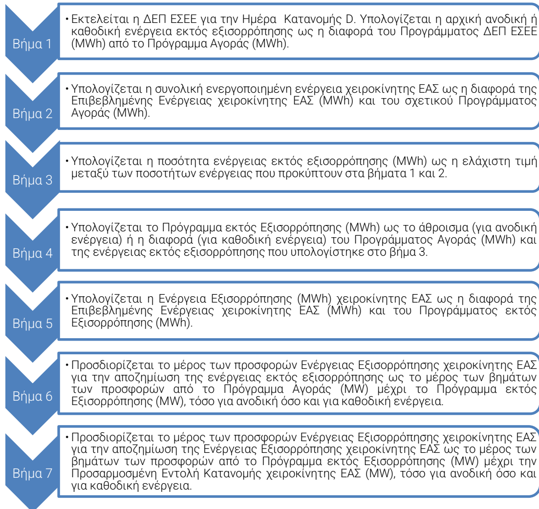
Σχήμα 3 Διαδικασία υπολογισμού της ενέργειας εκτός εξισορρόπησης για τις Κατανεμόμενες Μονάδες Παραγωγής και για τα Χαρτοφυλάκια Κατανεμόμενων Μονάδων ΑΠΕ Ελεγχόμενης Παραγωγής
