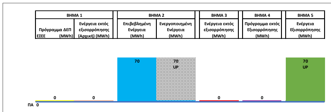
Σχήμα 23 Περίπτωση χαρακτηρισμού του συνόλου της ενεργοποίησης ως Ενέργεια Εξισορρόπησης (μηδενική ενέργεια εκτός εξισορρόπησης) - Βήματα 1-5
