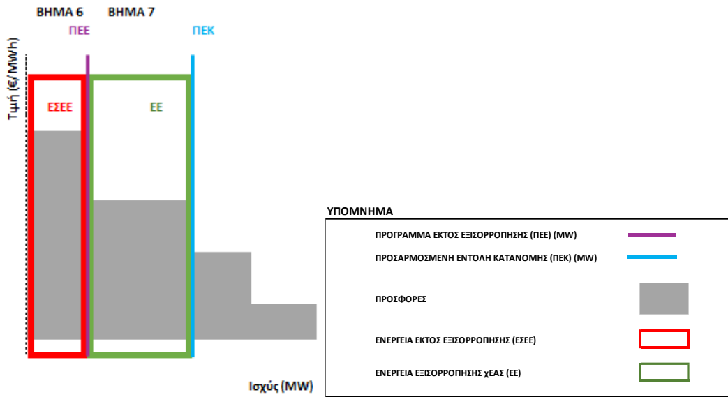
Σχήμα 8 Σχηματική αναπαράσταση των βημάτων 6-7 της μεθοδολογίας για καθοδική ενεργοποιημένη ενέργεια χειροκίνητης ΕΑΣ
