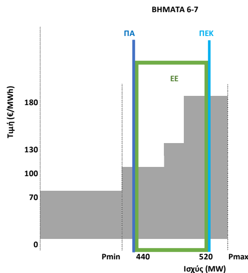
Σχήμα 20 Διάκριση ποσοτήτων στην ανοδική προσφορά χειροκίνητης ΕΑΣ - Βήματα 6-7
