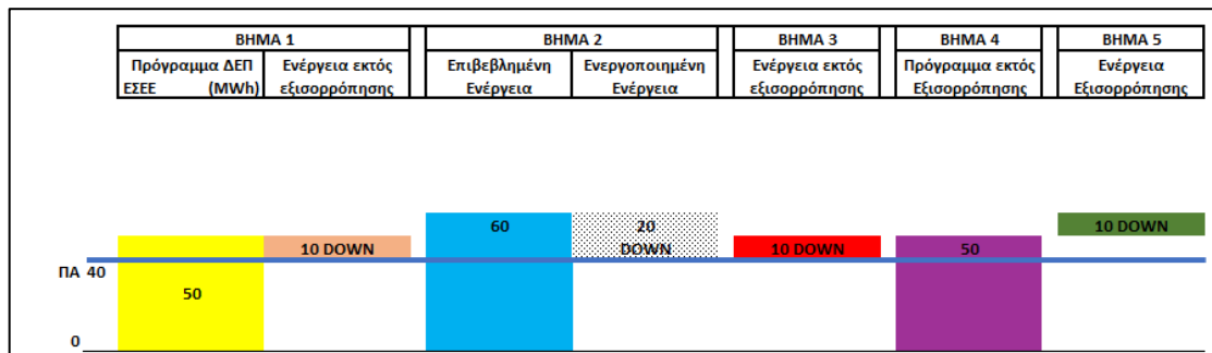
Σχήμα 36 Παράδειγμα με καθοδική ενεργοποιημένη ενέργεια χειροκίνητης ΕΑΣ για Χαρτοφυλάκιο Κατανεμόμενου Φορτίου σε λειτουργία άντλησης- Βήματα 1-5
