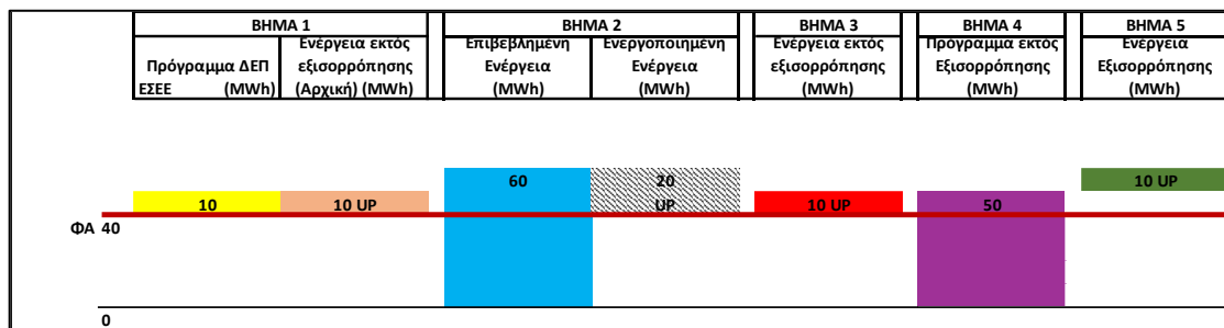
Σχήμα 26 Παράδειγμα με ανοδική ενεργοποιημένη ενέργεια για Χαρτοφυλάκια Κατανεμόμενων Μονάδων ΑΠΕ Μη Ελεγχόμενης Παραγωγής - Βήματα 1-5
