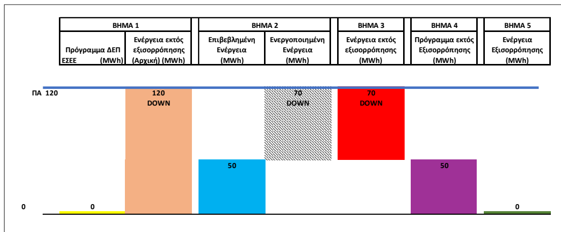
Σχήμα 21 Περίπτωση χαρακτηρισμού του συνόλου της ενεργοποίησης ως ενέργεια για σκοπούς εκτός εξισορρόπησης (μηδενική Ενέργεια Εξισορρόπησης χειροκίνητης ΕΑΣ) - Βήματα 1-5
